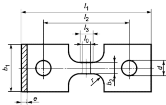
Рисунок 1 - Образец типа 3
